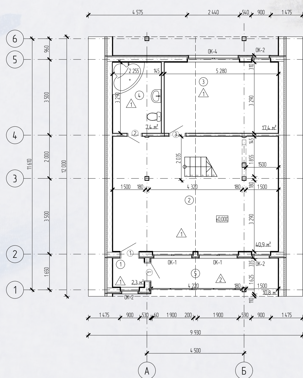
План 1-го этажа А-фрейма
