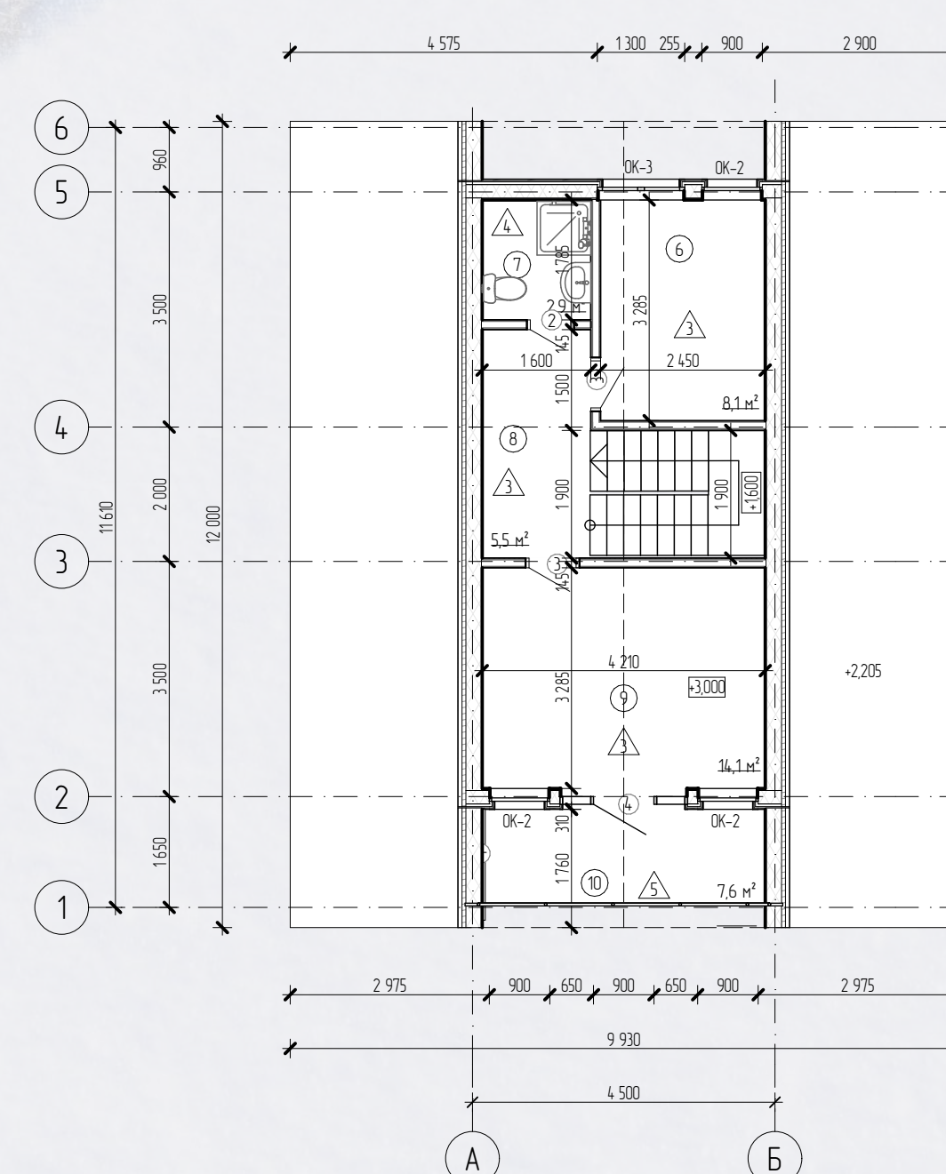
План 2-го этажа А-фрейма
